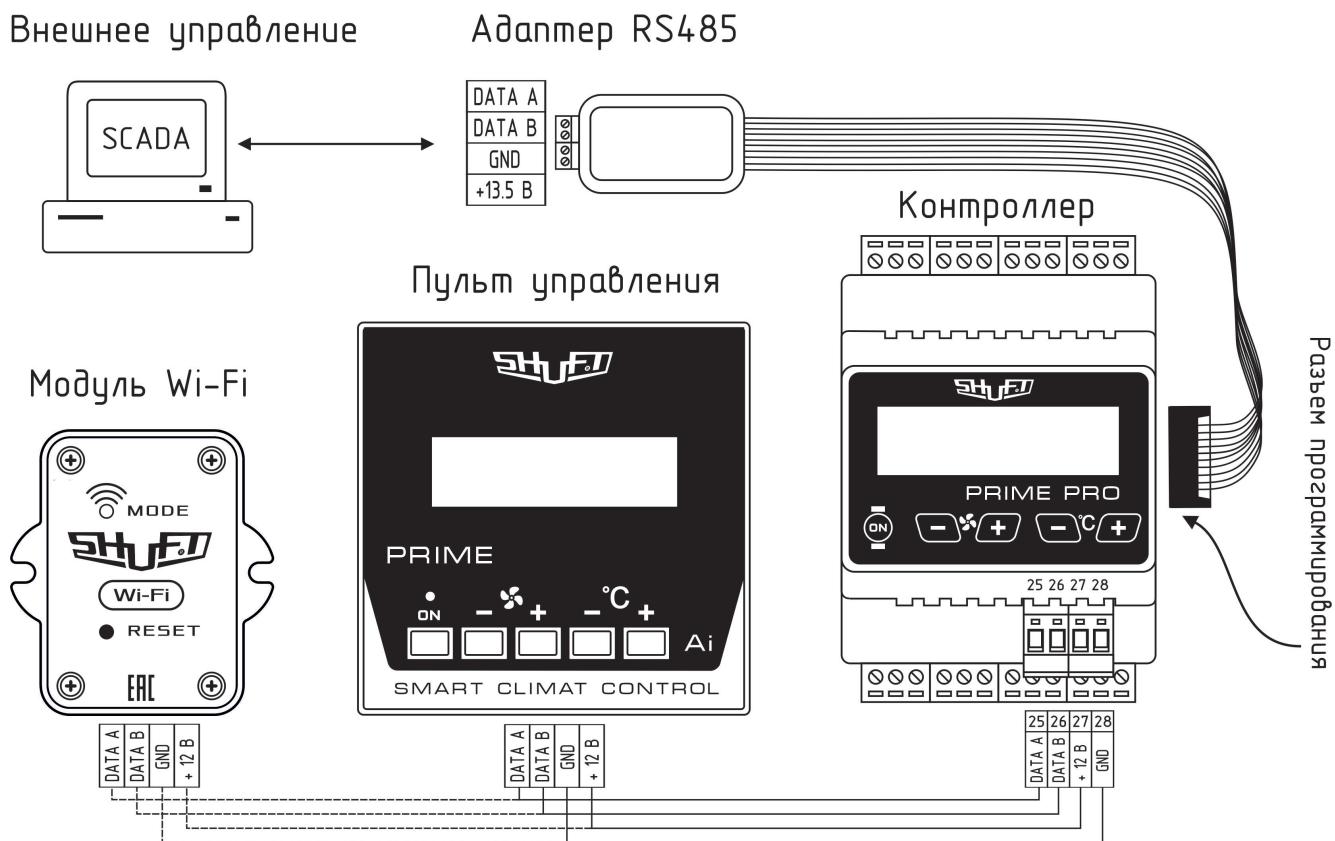
Рис. 2.3 Подключение средств ДУ + SCADA
