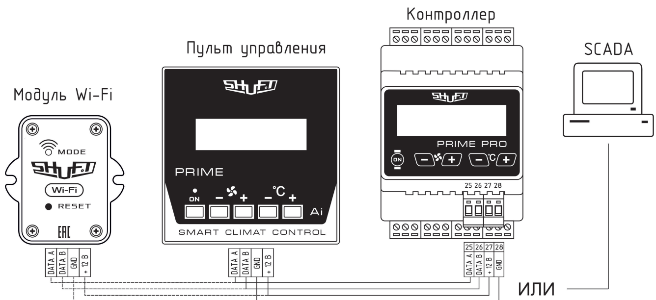
Рис. 2.2 Подключение средств ДУ
