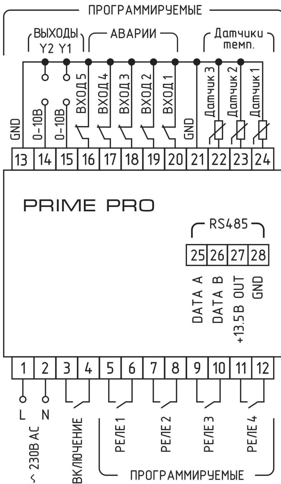
Рис. 2.1 Назначение клемм контроллера.
