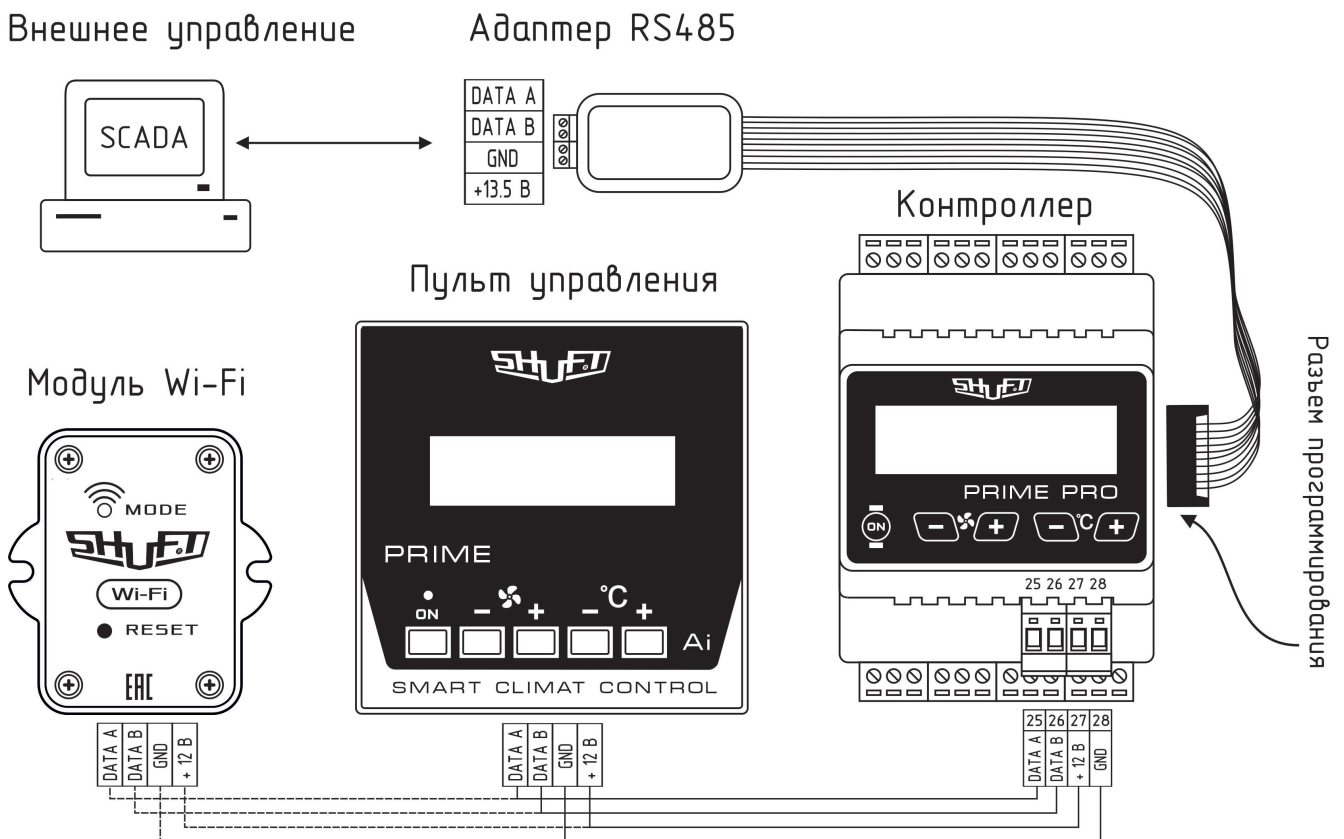
Рис. 6.4 Подключение внешних средств ДУ + SCADA
