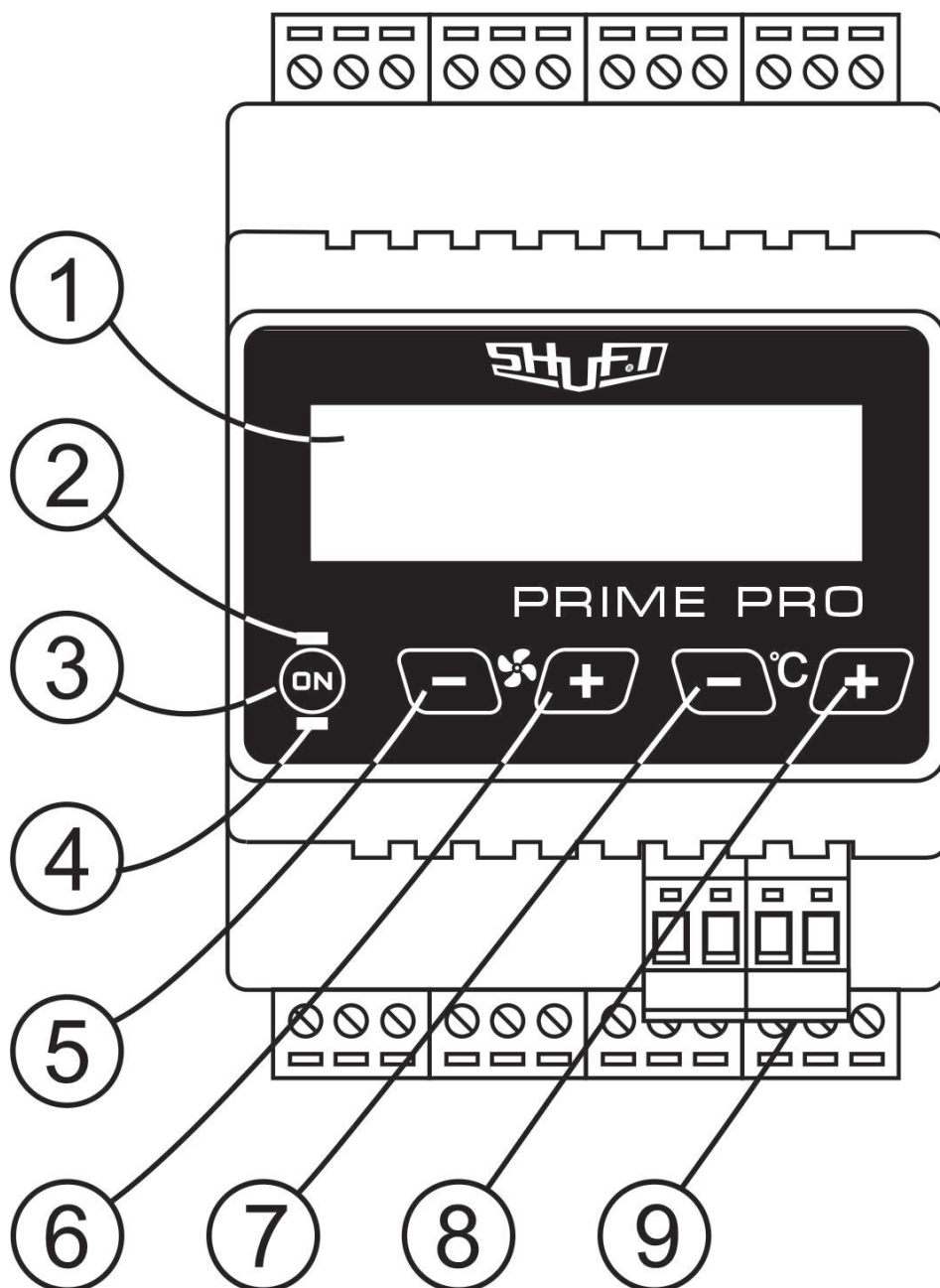
Рис. 1. Основные элементы контроллера
