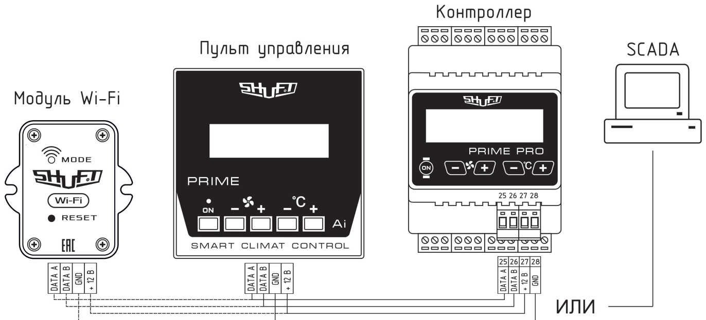
Рис. 6.3 Подключение внешних средств ДУ
